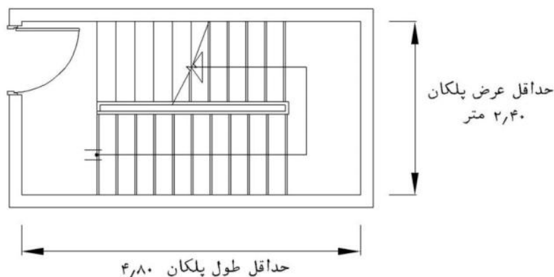
شکل ۳-۴-۳- ابعاد پلکان
